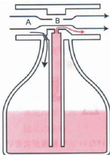
動作原理
