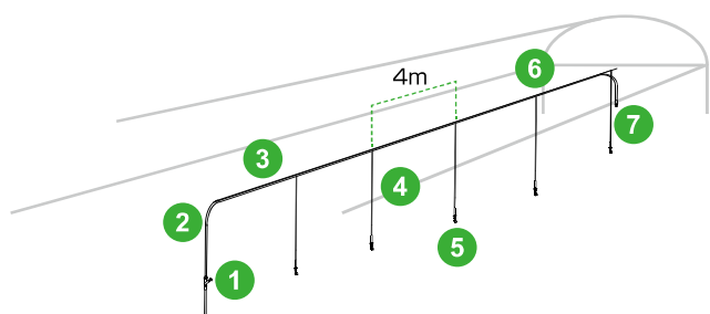
図13 ブルーベリー養液ドリップかん水システム配管例
