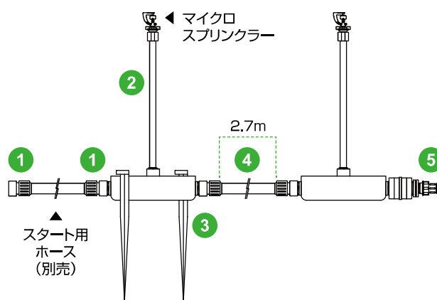
図16 プレート式配管例
