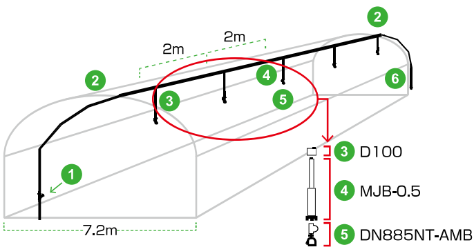
図02 ポリ式配管例
