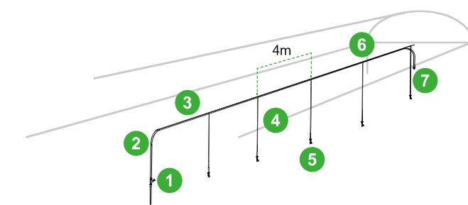
図12 サクランボ雨よけハウス配管例
