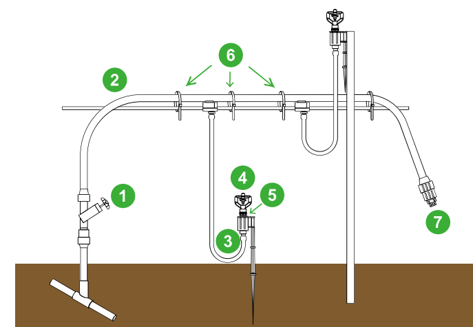
図07 棚配管例
