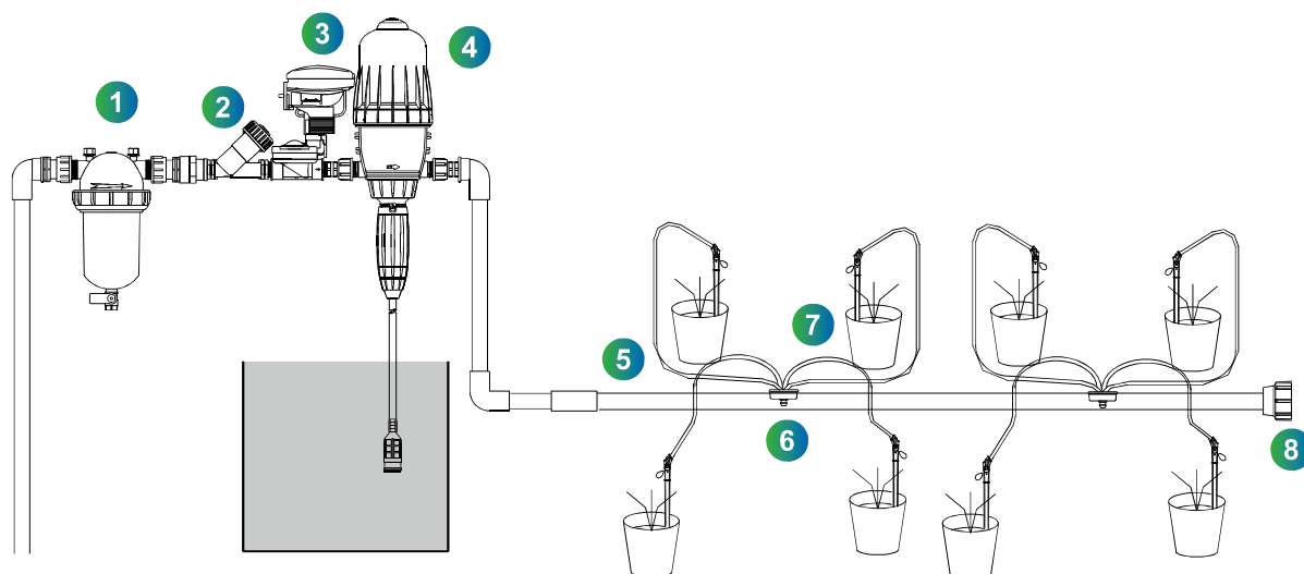
図22 チューブ付きマルチアダプター4分岐によるドリップファーターゲーション 配管例
