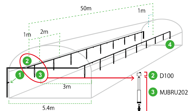
図04 ポリ式配管例
