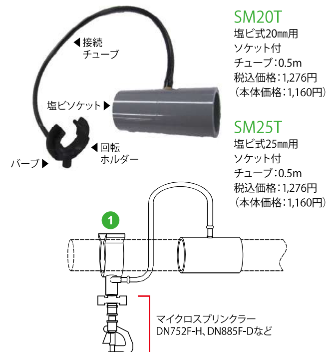
図05 塩ビ式セット
