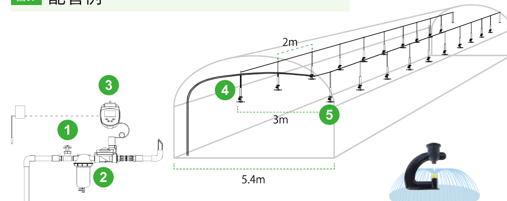
図09 配管例
