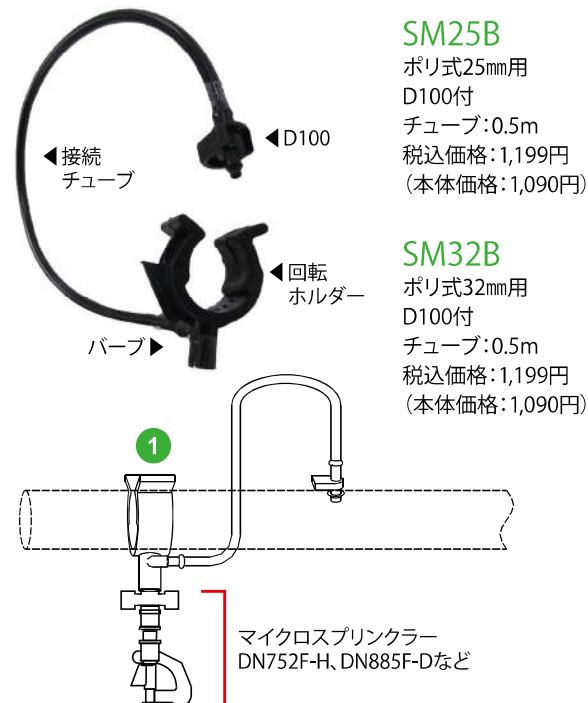
図06 ポリ式セット
