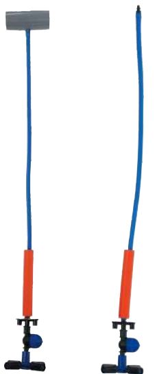
【塩ビ式配管直付用資材】
