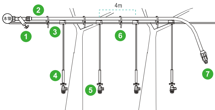
図11 リンゴ 新わい化ドリップかん水システム配管例
